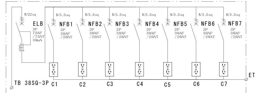
結線図
