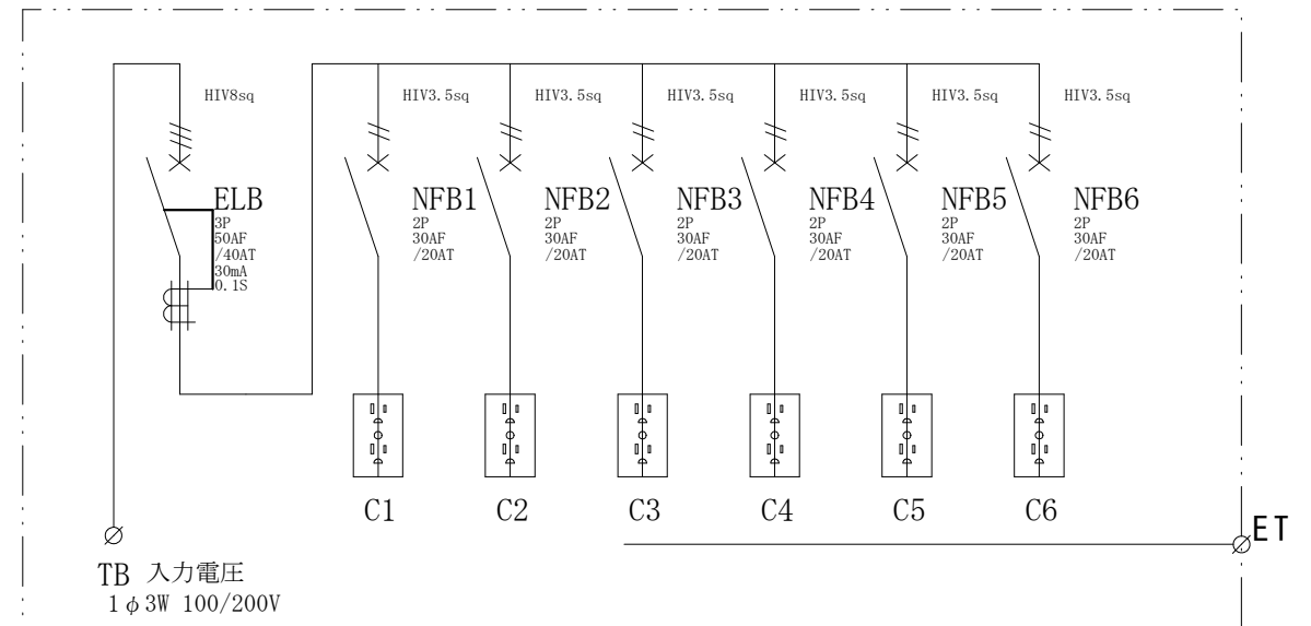
結線図
