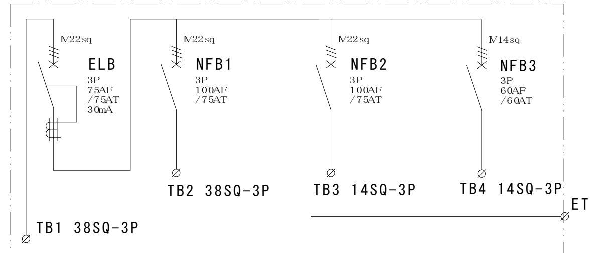
結線図
