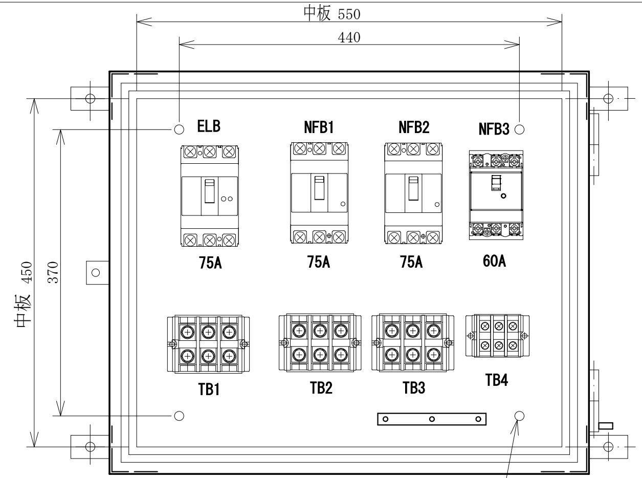
配置図
