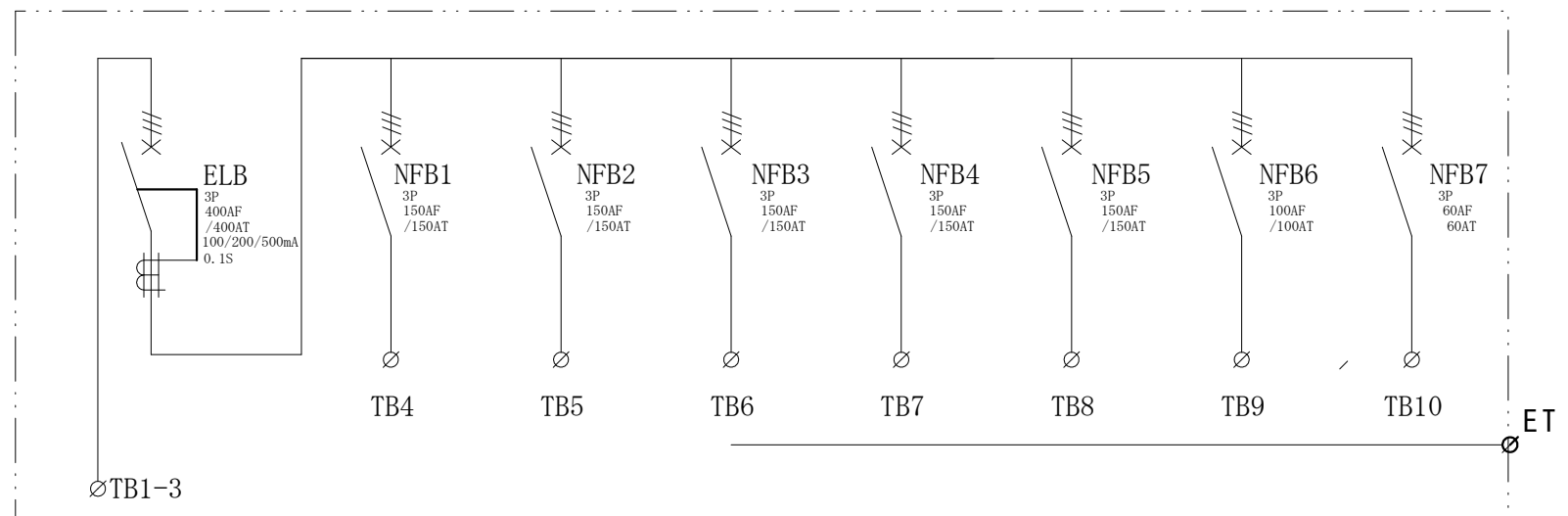
結線図
