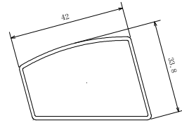
A-A断面 S = 1 : 1
