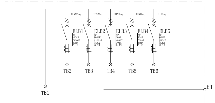
結線図
