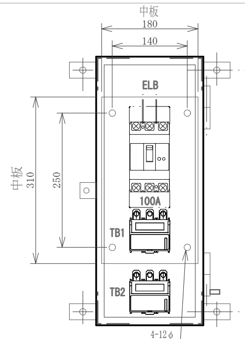
配置図
