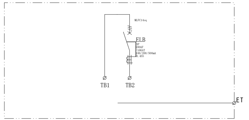
結線図
