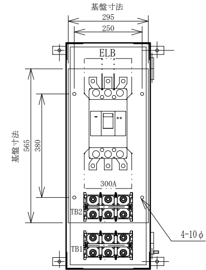
配置図
