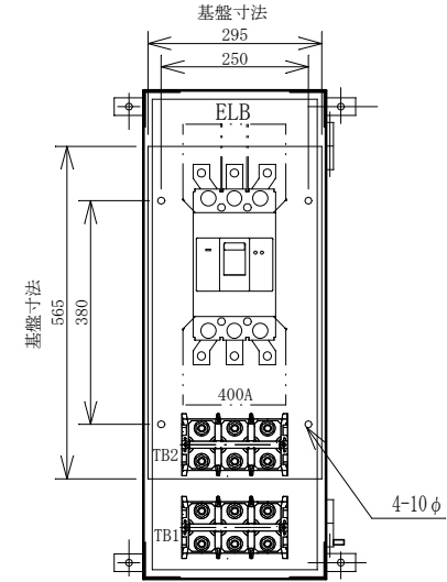
配置図
