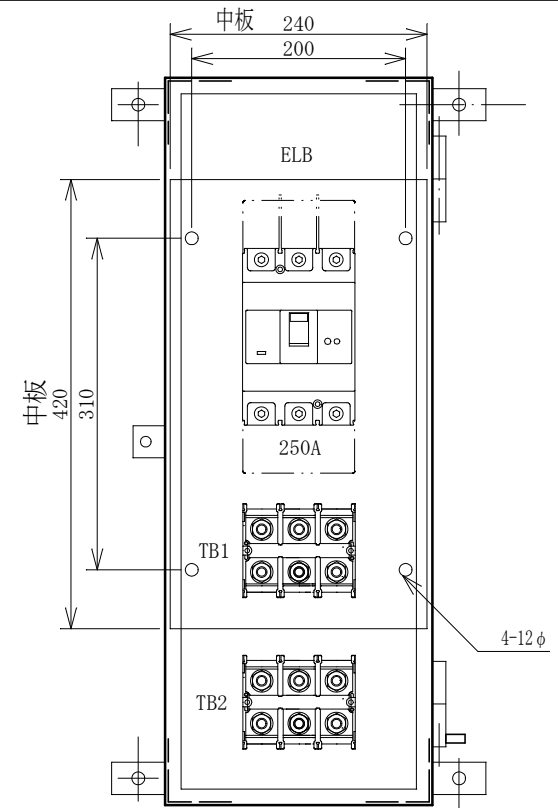
配置図 結線図
