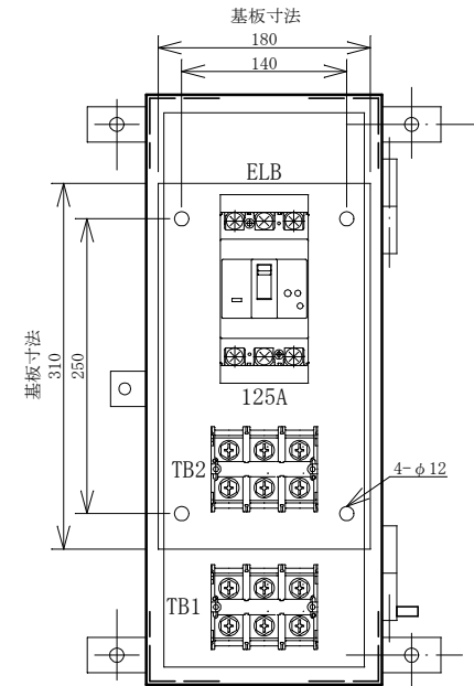
配置図
