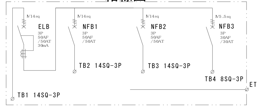
結線図
