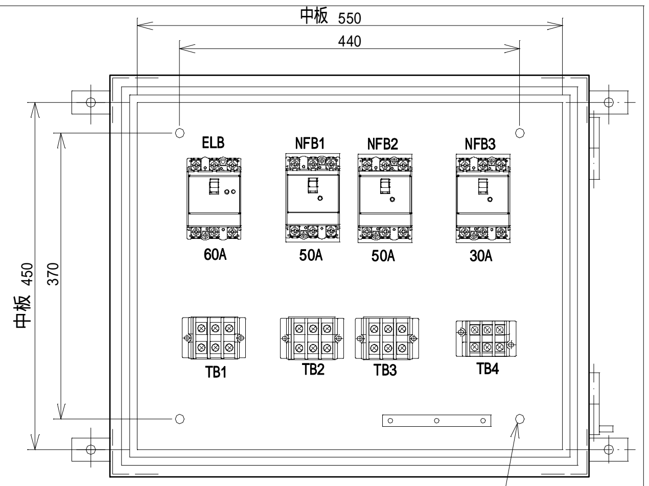
配置図
