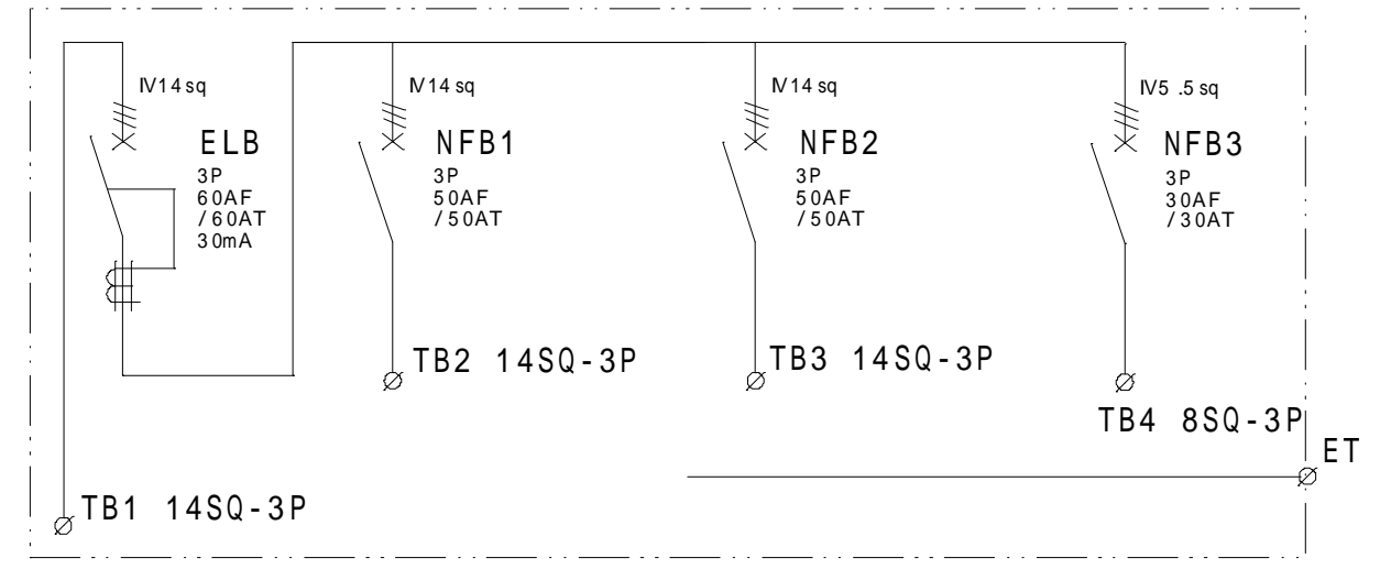
結線図
