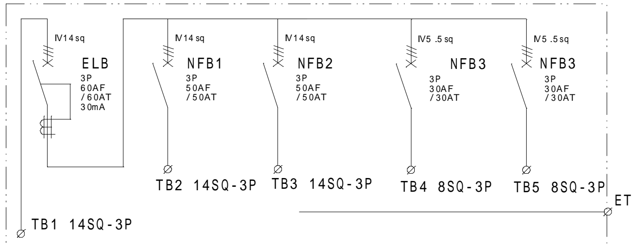
結線図
