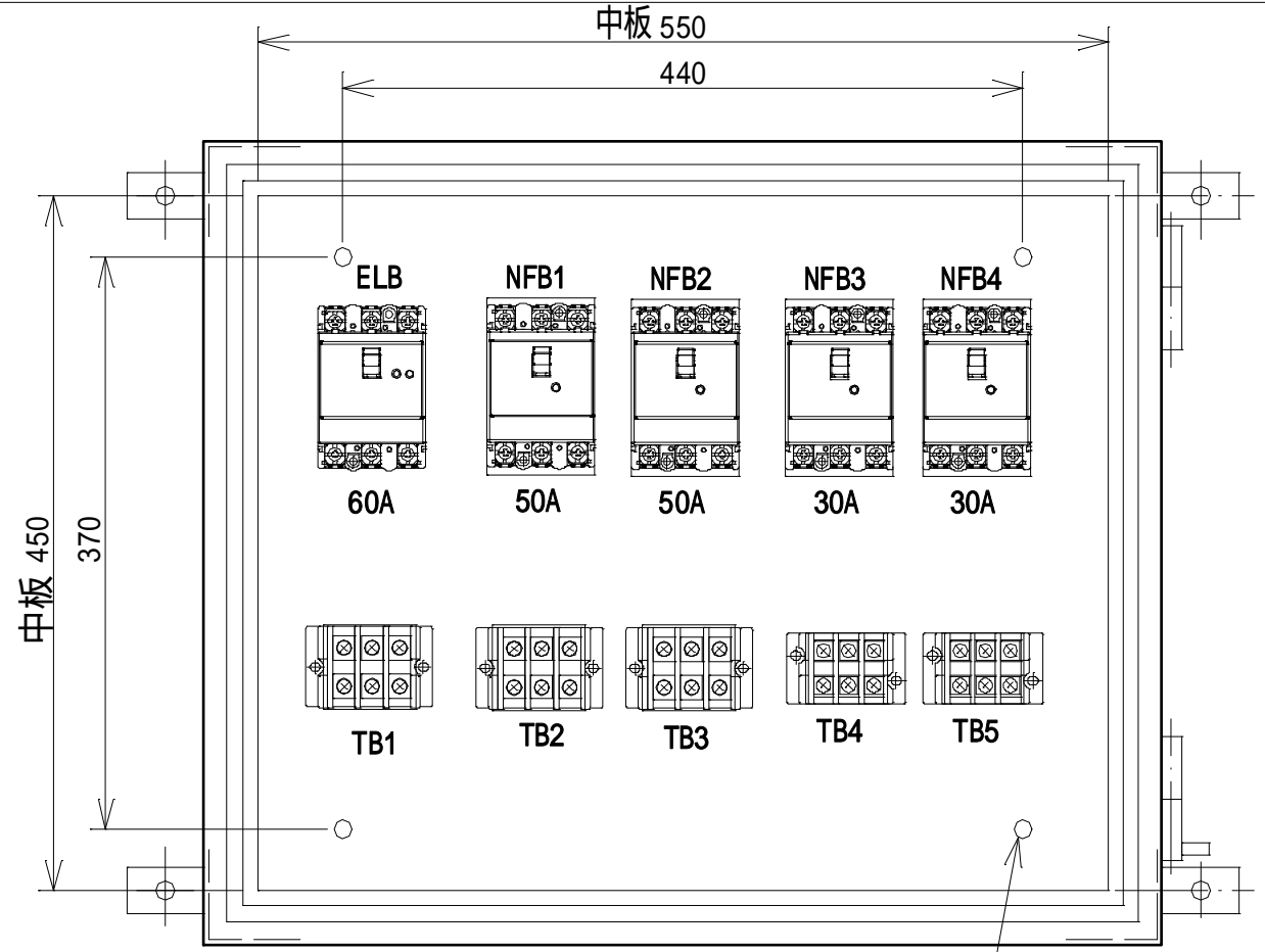
配置図
