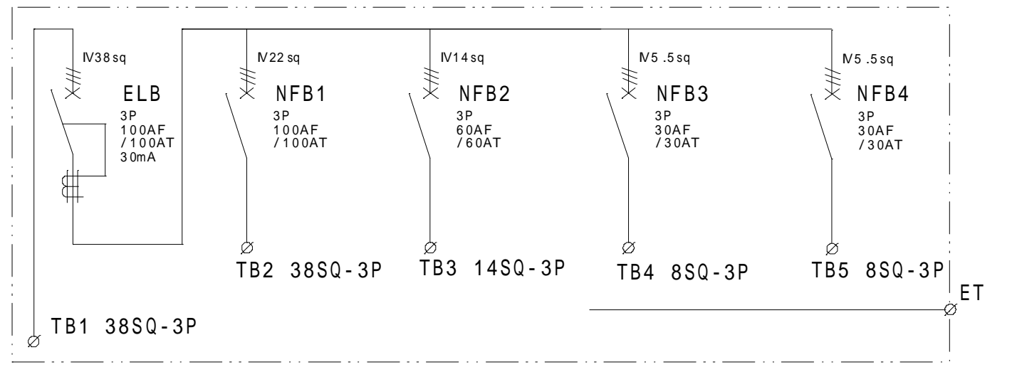
結線図
