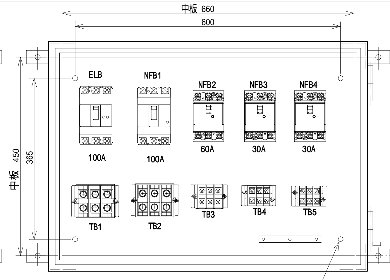
配置図
